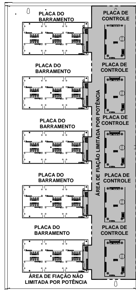
Ilustração 3: Separação da Fiação do Compartimento com N/P 10-2777-09 Conjunto de Controle de Relés
