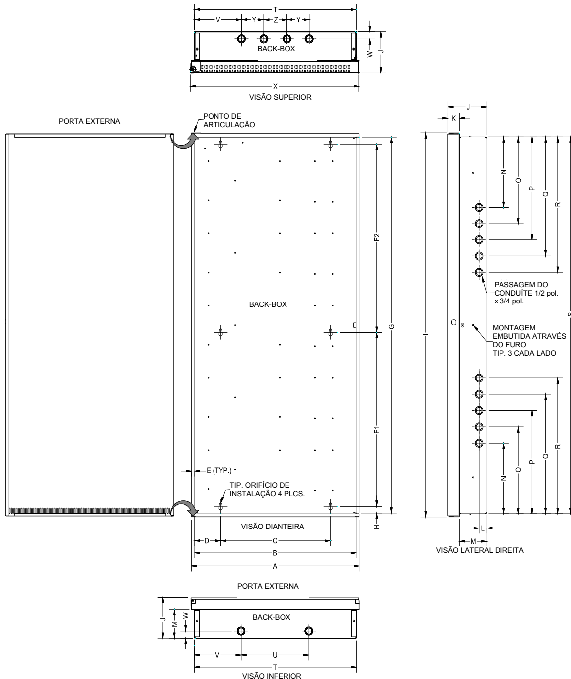
Ilustração 4: Compartimento de 5 Slots
