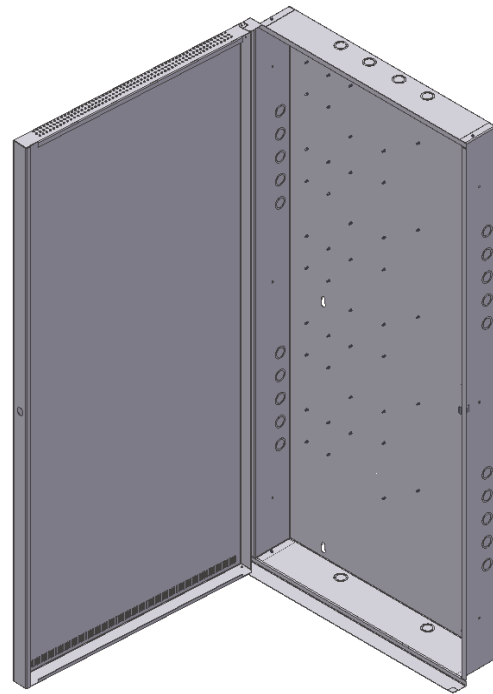
Ilustração 1: Compartimento de Equipamento Remoto de 5 Slots
