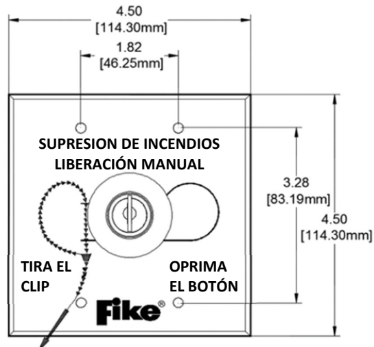
Vista frontal del interruptor de desbloqueo manual
