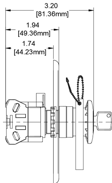
Vista lateral del interruptor de desbloqueo manual
