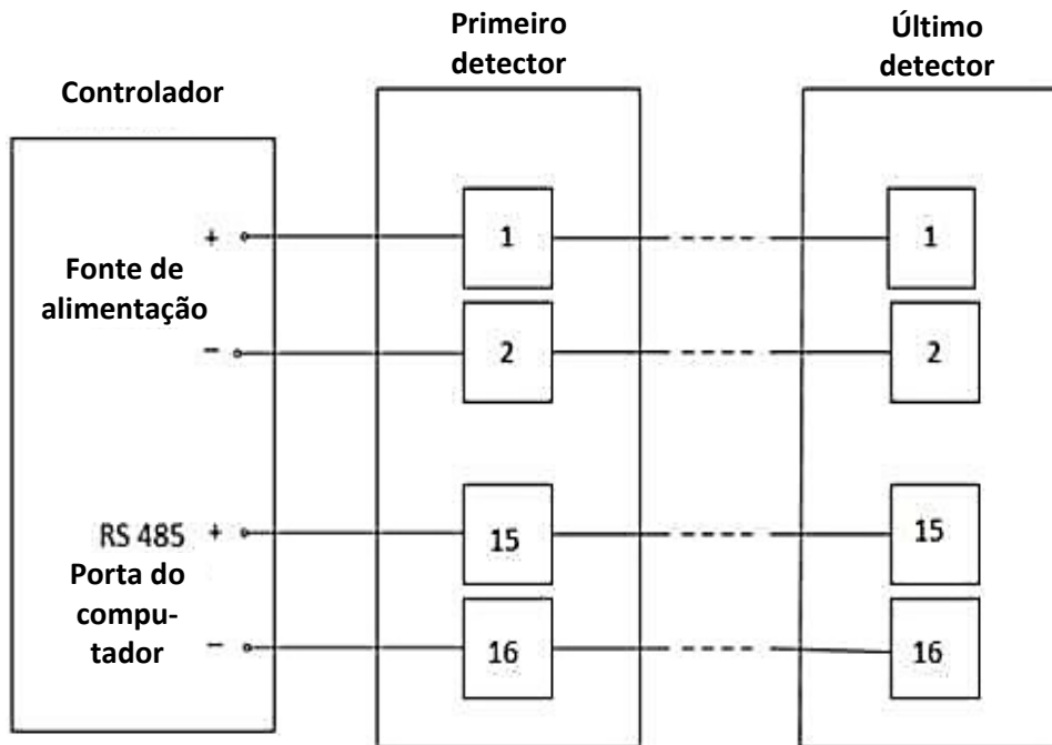
Figura 8: Rede RS-485
