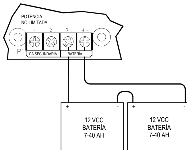
Figura 35 Cableado de batería de reserva
