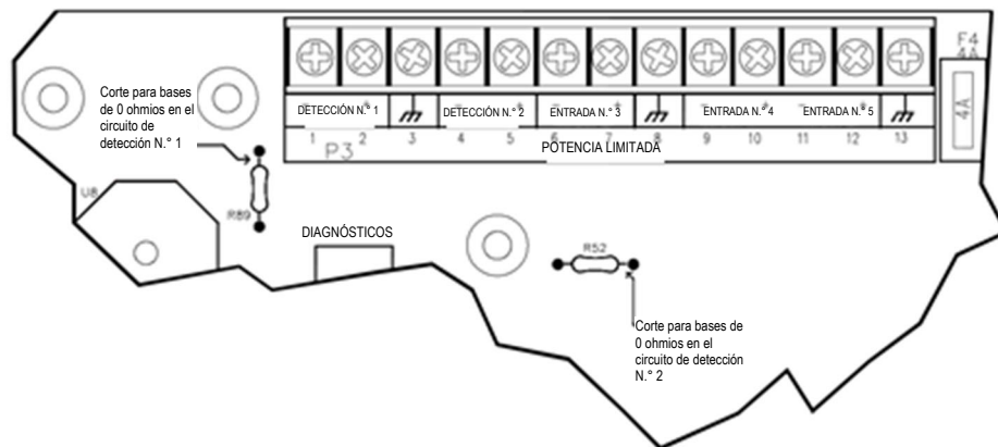
Figura 38 Ubicaciones de puentes de 0 \Omega
