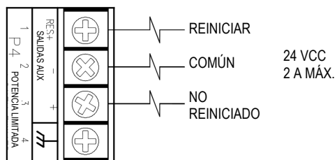
Figura 39 Cableado del circuito de alimentación auxiliar
