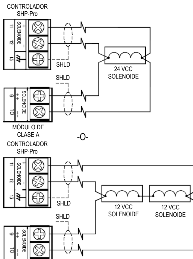
Figura 46 Cableado clase A de salida del solenoide
