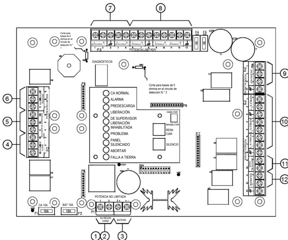
Figura 13 Controlador SHP-Pro
