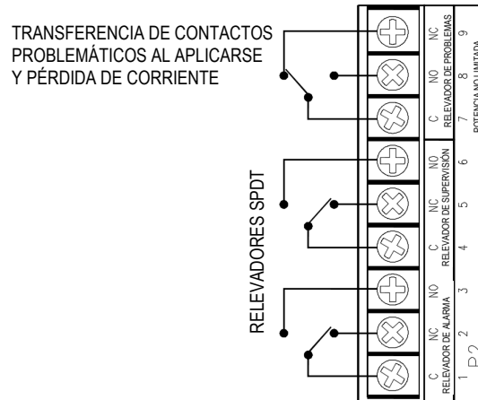
Figura 36 Cableado de relevador común (mostrado con corriente aplicada)
