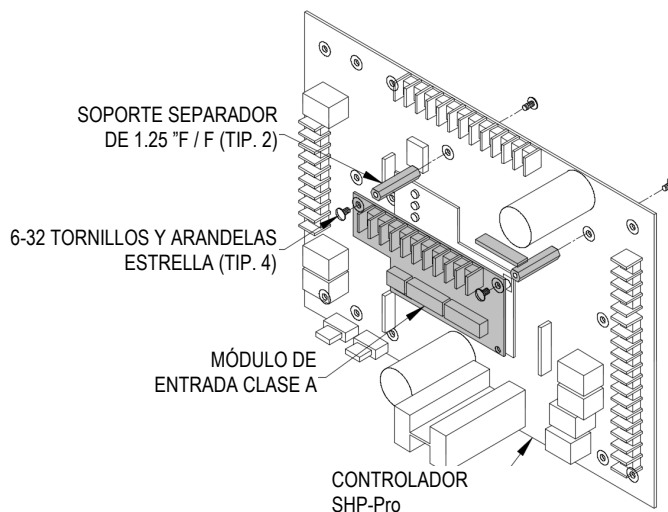
Figura 26 Ubicaciones opcionales de montaje de los módulos
