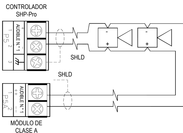
Figura 44 Cableado clase A de las salidas audibles N.º 1 a N.º 3
