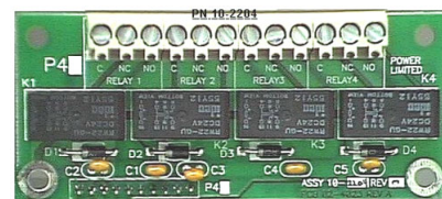
Figura 6 Módulo de relevador CRM4
